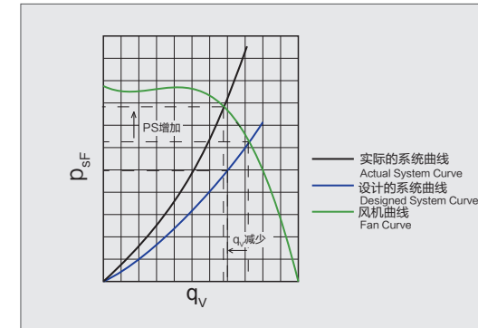
图5 系统阻力曲线的变化——风量减少
