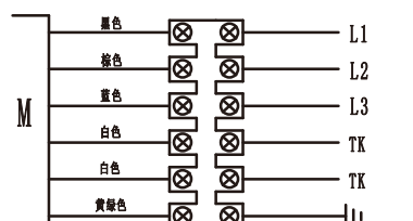
外转子风机三相接线图
