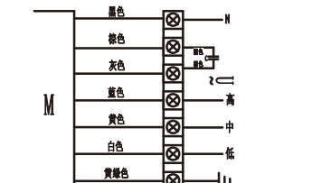
外转子风机单相三速接线图
