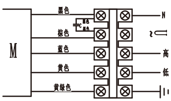
外转子风机单相双速接线图
