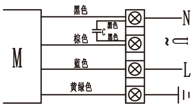
外转子风机单相接线图
