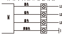
外转子风机三相接线图
