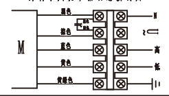
外转子风机三相三速接线图
