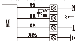
外转子风机单相接线图
